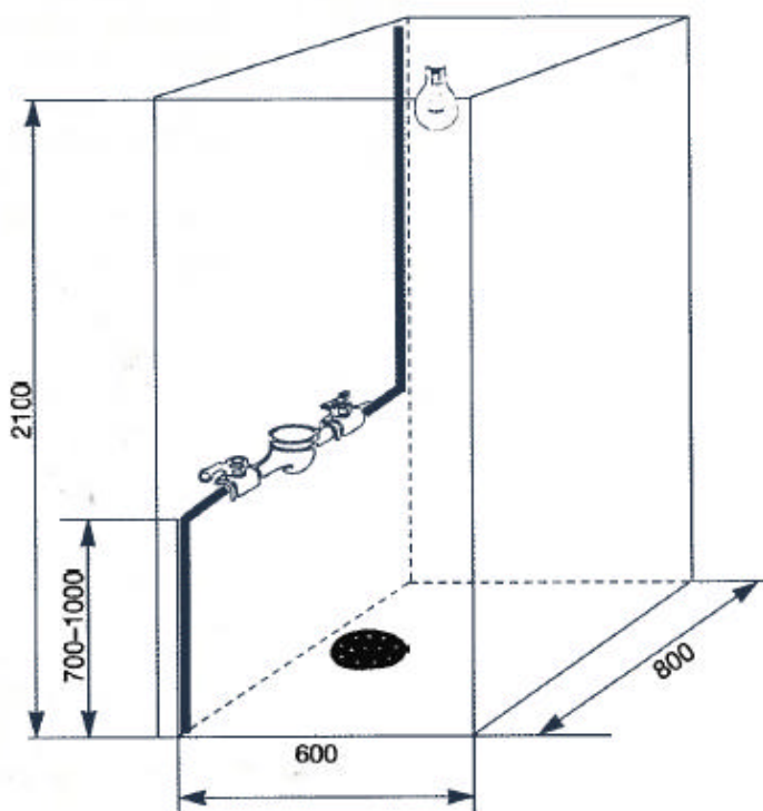
Figur 2: För att komma åt vattenmätaren för avläsning eller service måste det finnas ett fritt utrymme runt mätaren enligt denna figur. Alla mått i mm.
