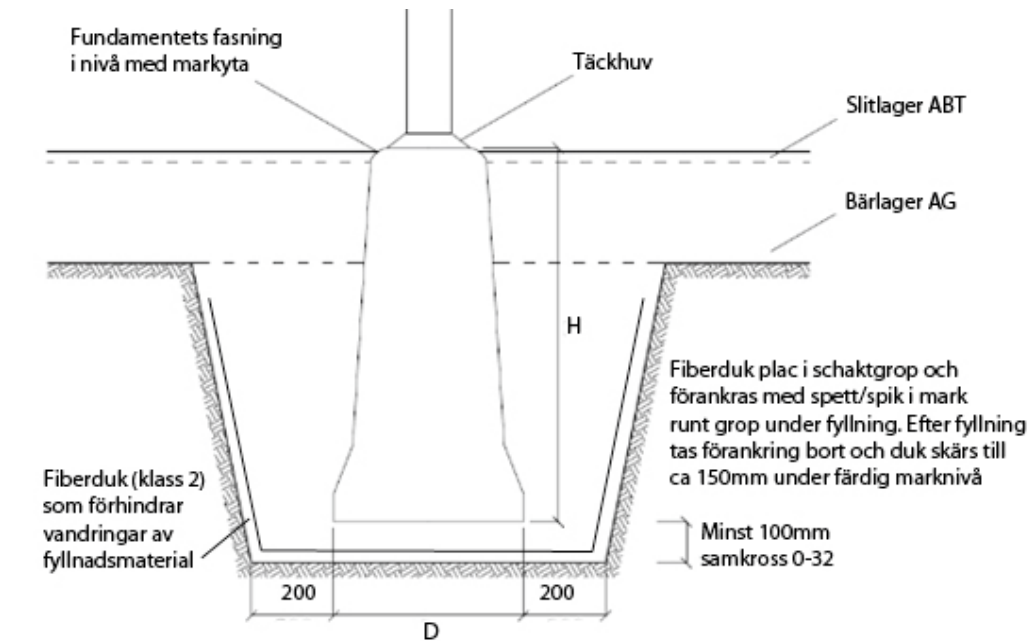
Bild 1 Fundament i asfalt- eller plattytta
