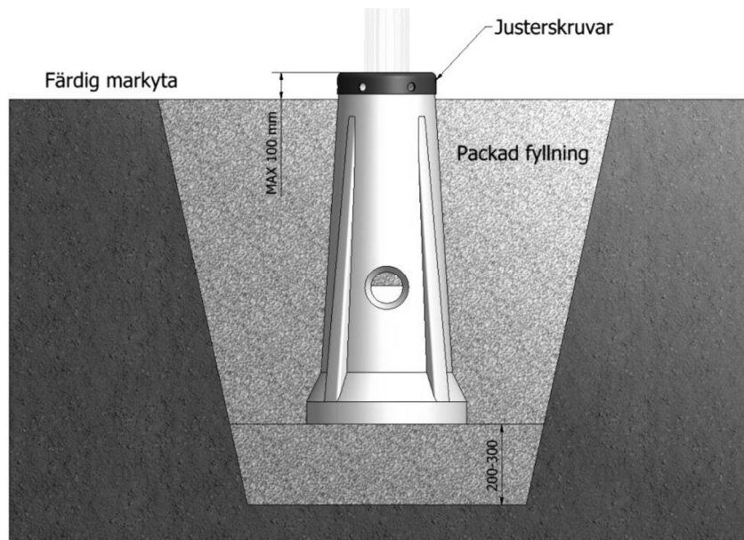
Bild 3 Fundament för absorbentstolpe
