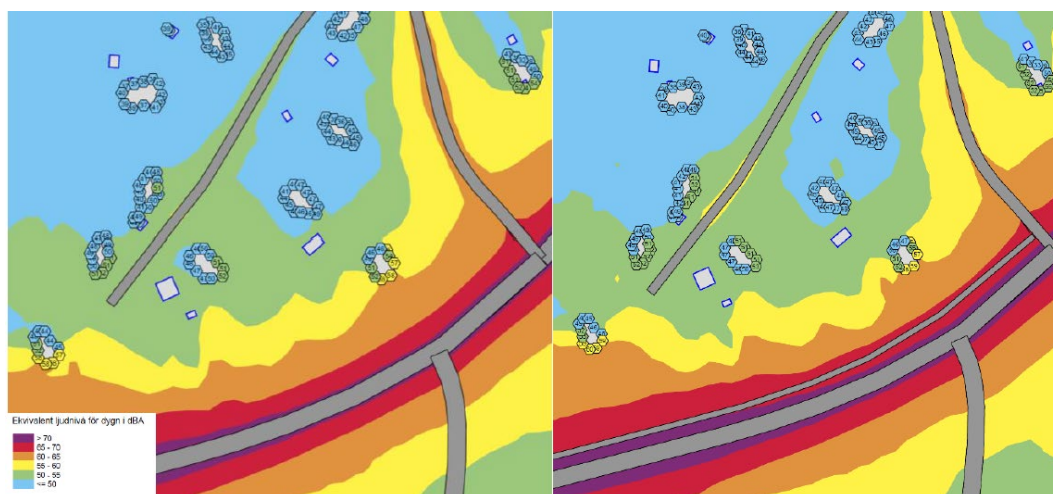
Figur 16. Dygnsekvivalent ljudnivå från Saltarövägen för befintlig bebyggelse i Norra Kopparmora med sommartrafik år 2023 (vänster) respektive 2040 (höger) som inkluderar GC-bana.
