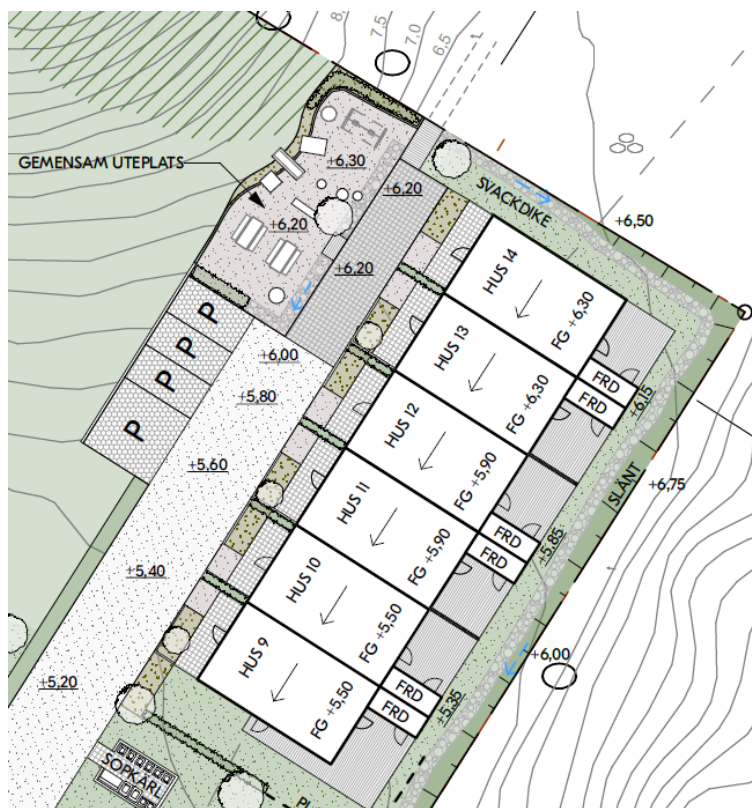
Figur 28. Exempel gårdsutformning, marktbehandling, Blooc AB.
