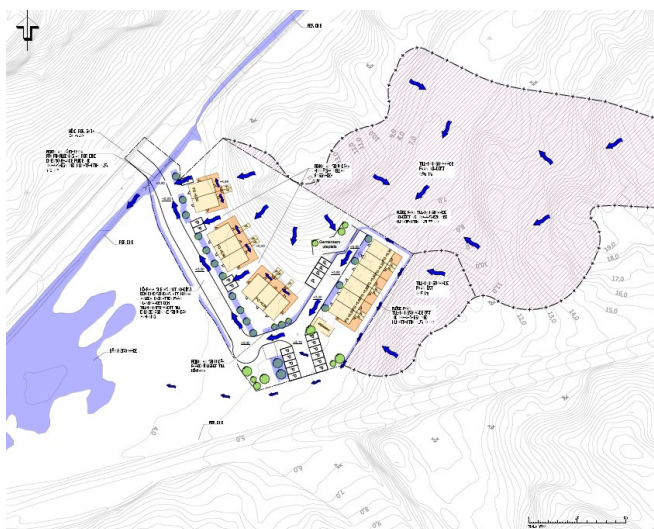
Figur 20. Bilden visar sekundära rinnvägar inom planområdets kvartersmark, vid skyfall, Marktema (2021).
