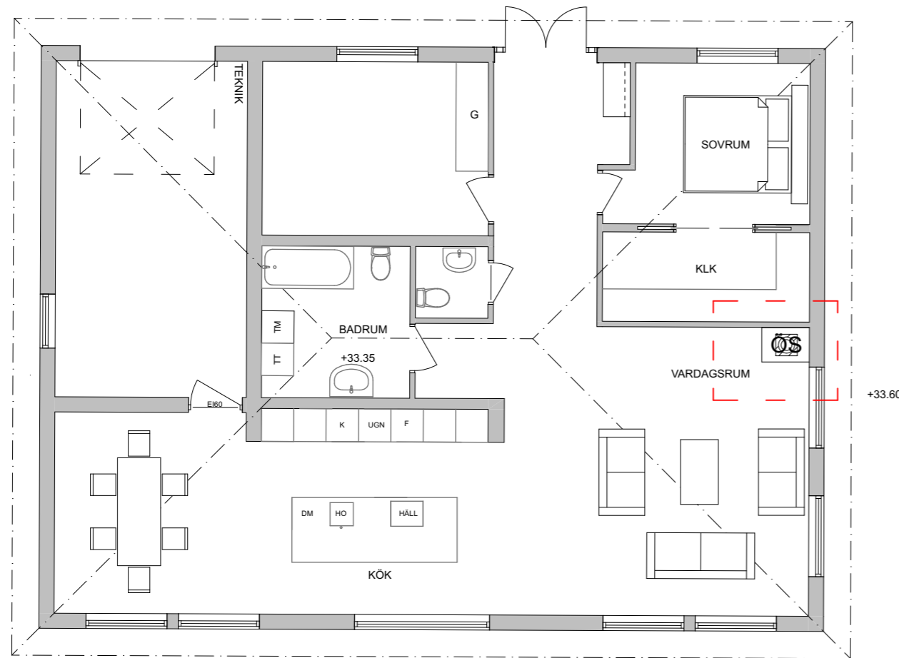
ange plan 1:100
